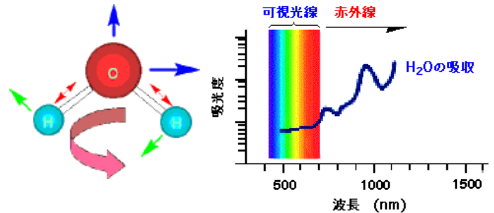
水分子の運動
