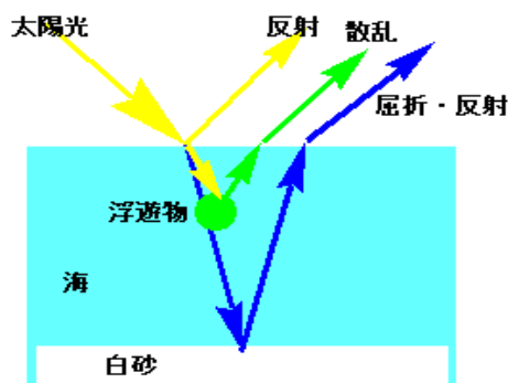
海面での反射、浮遊物での散乱、海底での反射
