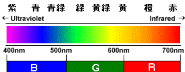
太陽光のスペクトル
