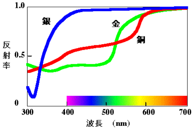
金、銀、銅の反射率と波長依存性
