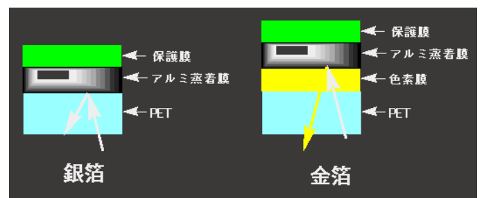
銀箔と金箔の構造
