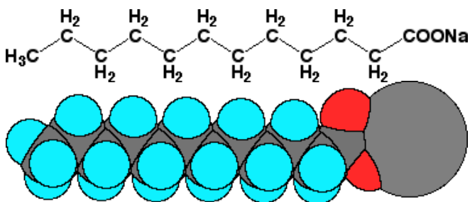
ラウリン酸ナトリウムと分子モデル
