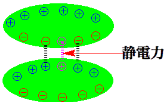
van der Waals 力
