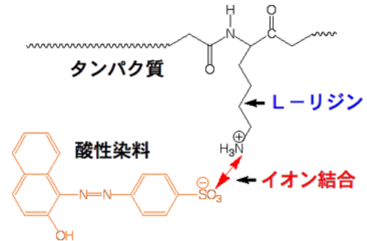
ウールや絹と酸性染料のイオン結合
