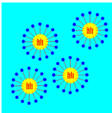
せっけんが油を溶かした図
