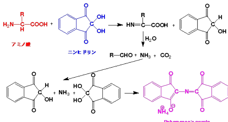
アミノ酸とニンヒドリンの反応でルーエマン紫の色素ができる
