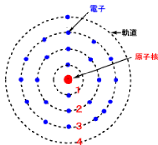
クロム原子の電子軌道
