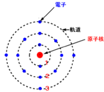
Al 原子の電子配置
