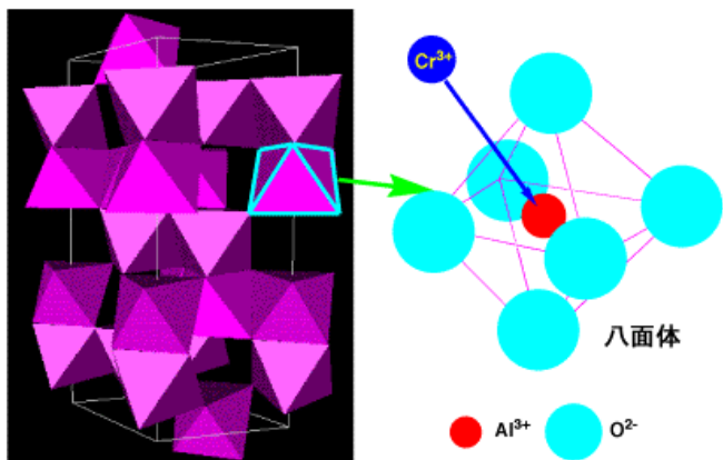
\alpha -アルミナ( Al_2O_3 )の結晶構造
