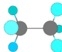
CH 3 -CH 3 エタン
