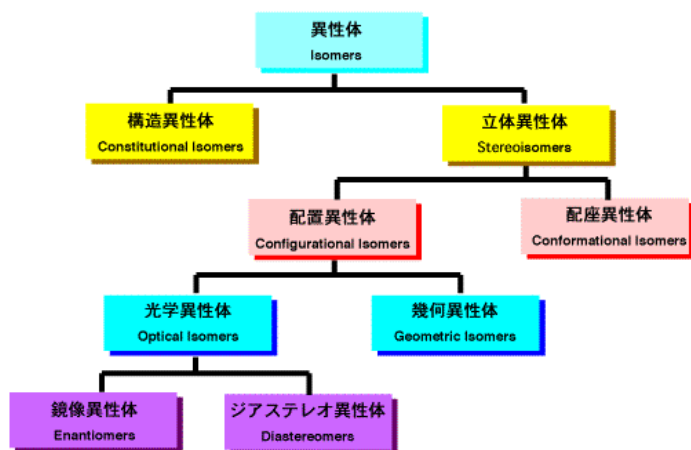
異性体の種類
