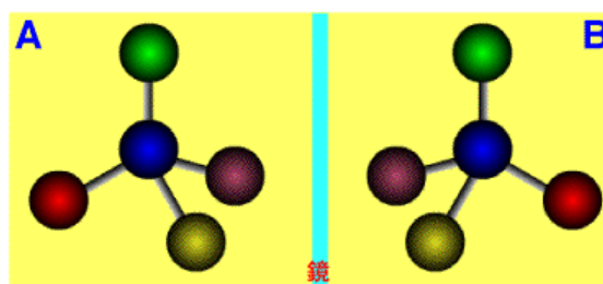
鏡像体：右と左は鏡に写した関係になっている
